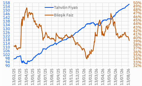
Kısa Vade DİBS (TRT100227T13)
