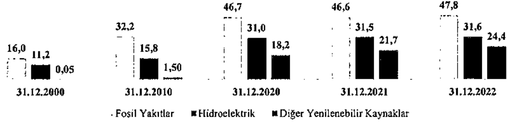
Grafik-7: Yıllar İtibarıyla Kurulu Gücün Kaynaklara Göre Dağılımı (GW) 11
