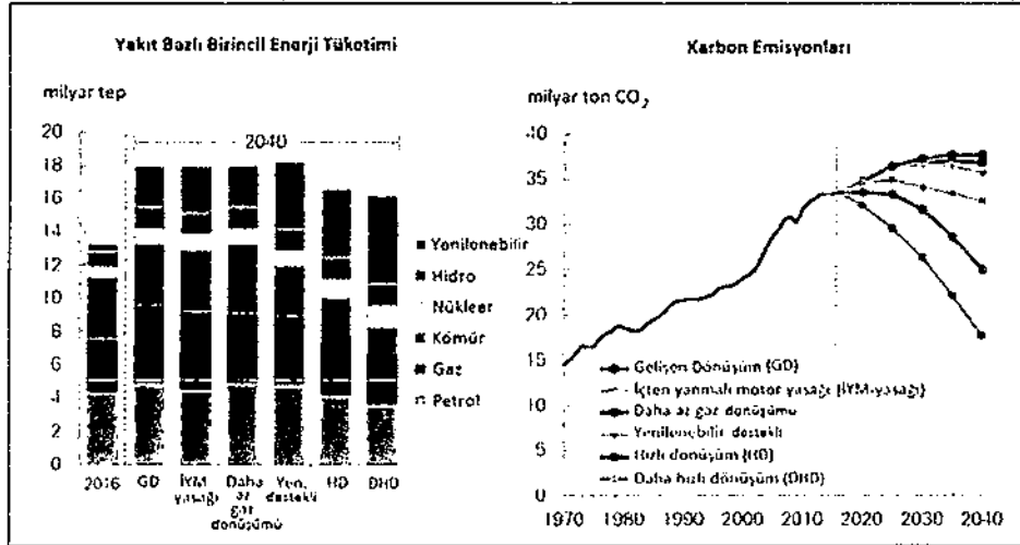
Grafik-2: 2040 yılına kadar Yakıt bazlı birincil enerji tüketimi ve karbon emisyonunun seyri projeksiyonu 6
