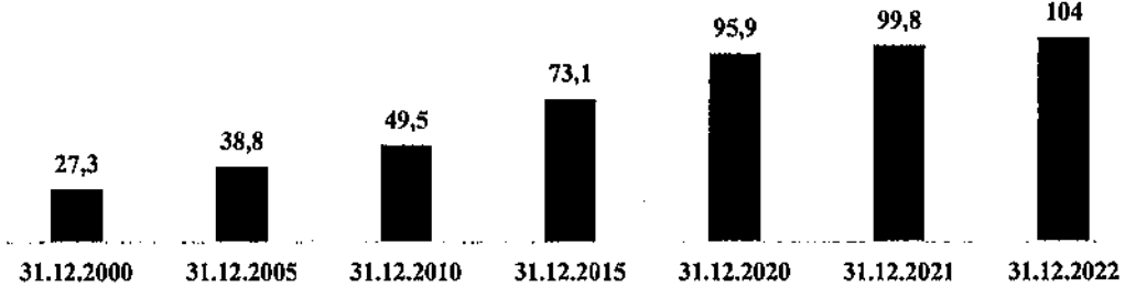
Grafik-6: Yıllar İtibarıyla Türkiye Elektrik Kurulu Gücü Gelişimi (GW) 10
